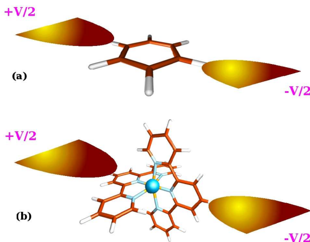
Bild 7: (a) Schematisches Bild eines einzelnen Benzol-Moleküls, welches über Tunnelbarrieren an zwei elektronische Reservoire angekoppelt ist. (b) Ein metallorganischer Komplex zwischen zwei Zuleitungen. Der Komplex besteht aus einem magnetischen Metallzentrum (z.B. Kobalt) und zwei zangenförmigen organischen Liganden, die über Thiol-Gruppen kovalent an Gold-Elektroden ankoppeln können. Referenzen: M.H. Hettler, W. Wenzel, M.R. Wegewijs, and H. Schoeller, Phys. Rev. Lett. 90, 076805 (2003); J. Park et al., Nature 417, 723 (2002).
